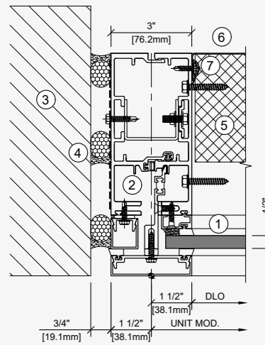
Jamb detail
