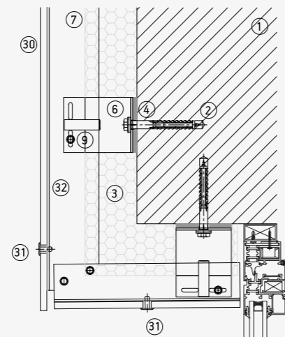
Dekton lintel
