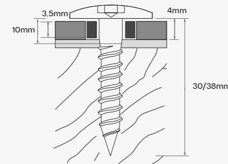
Fix point - Dekton 4 mm
