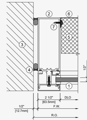
Jamb detail
