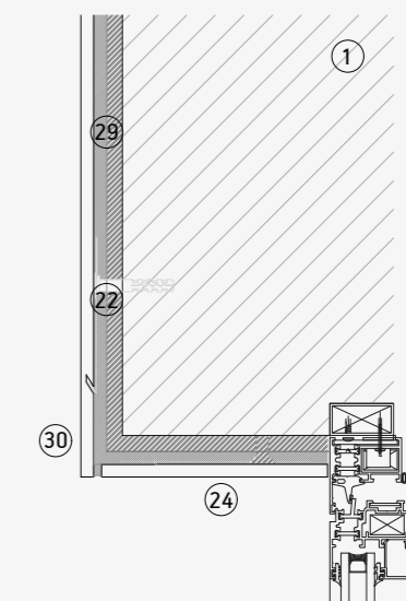
Dekton lintel
