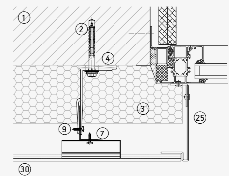
Metallic jamb
