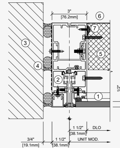
Jamb detail
