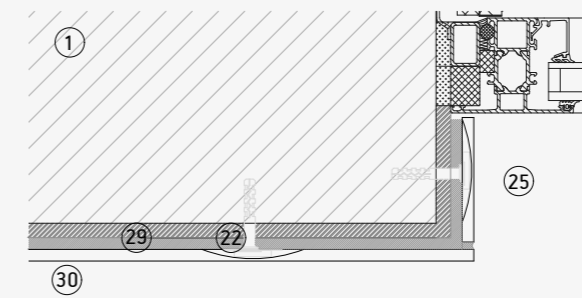
Dekton jamb
