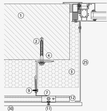
Metallic jamb
