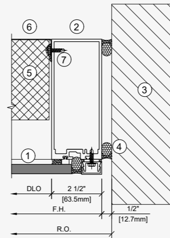
Jamb detail
