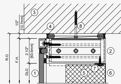
Top edge
