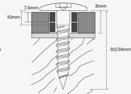
Fix point - Dekton 8 mm
