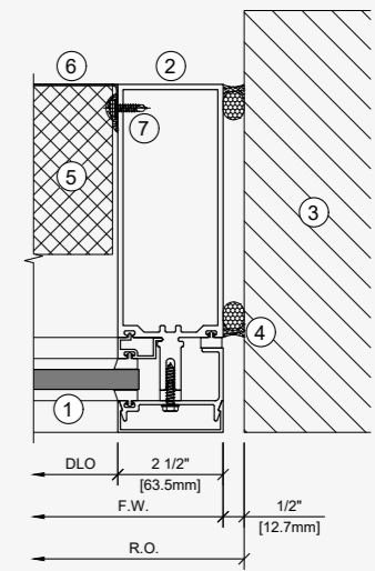
Jamb detail
