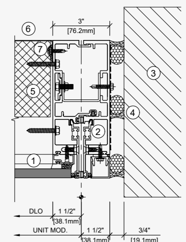
Jamb detail
